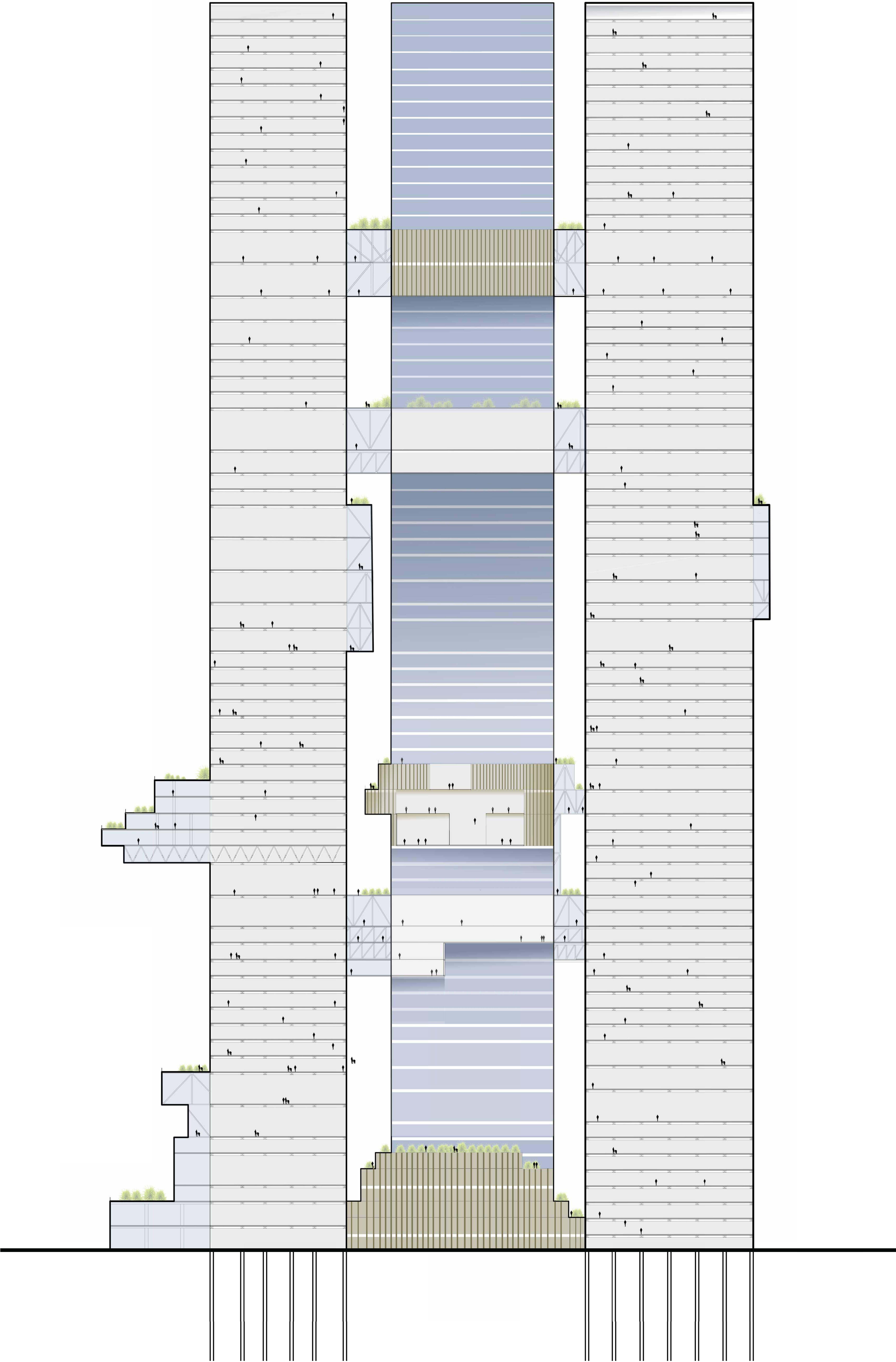
Section A-A
